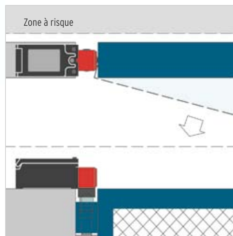
▼ D4NH, fixation à la porte.
