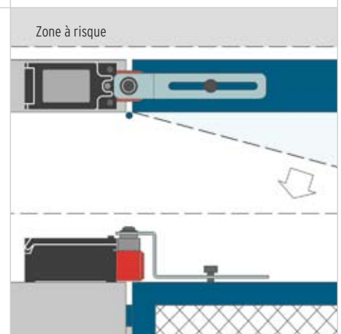
▼ D4NH, fixation dans l'axe du pivot.
