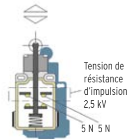
▼ Détails du mécanisme de rupture positive.
