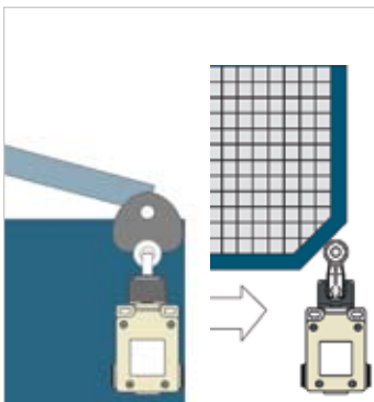
▼ Activation d'ouverture directe.
