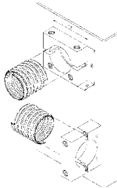
Système de fixation
